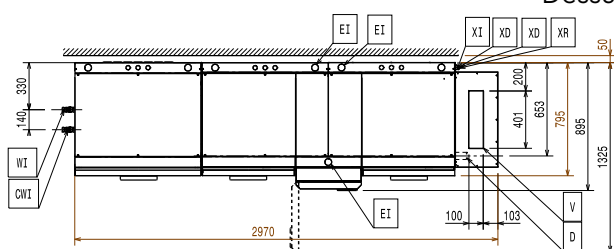
Dessus
